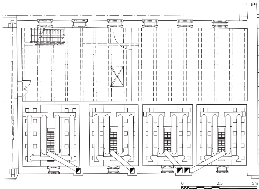
4.2 Výřez půdorysného plánu čtyřhvzdové sušárny chmele v Trnovanech u Žatce, č. p. 9, autoři: Jan Horák, David Skalický 2017.
