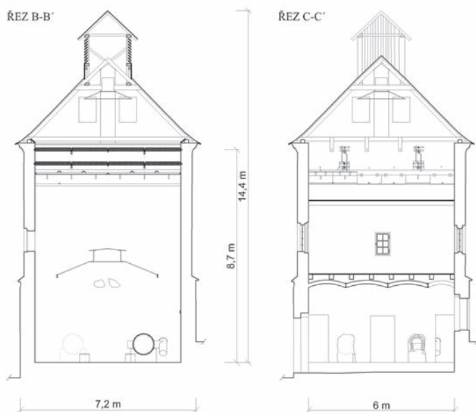
4.9 Příčné řezy sušárnou chmele v Siremi č. p. 5, autoři: Jan Horák, David Skalický 2017.
