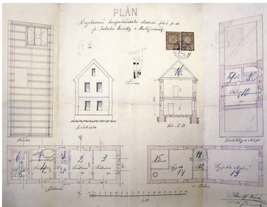
5.1 Plán obytného domu se sušárnou chmele v Mutějovicích č. p. 53, (SOA v Praze, SOKA Rakovník, Berní správa Rakovník, karton 42), kopie originálu: Renata Kuprová 2017.
