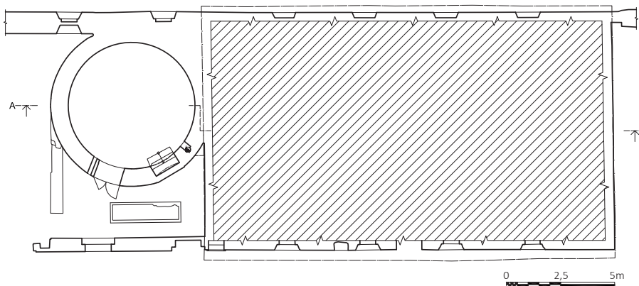
2.11 Půdorys 1. NP sušárny v Rybňanech, p. č. 10/3, autoři: Jan Horák, David Skalický 2018.
