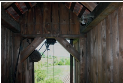
008 – Pohled elektrický na pohon vrátku
