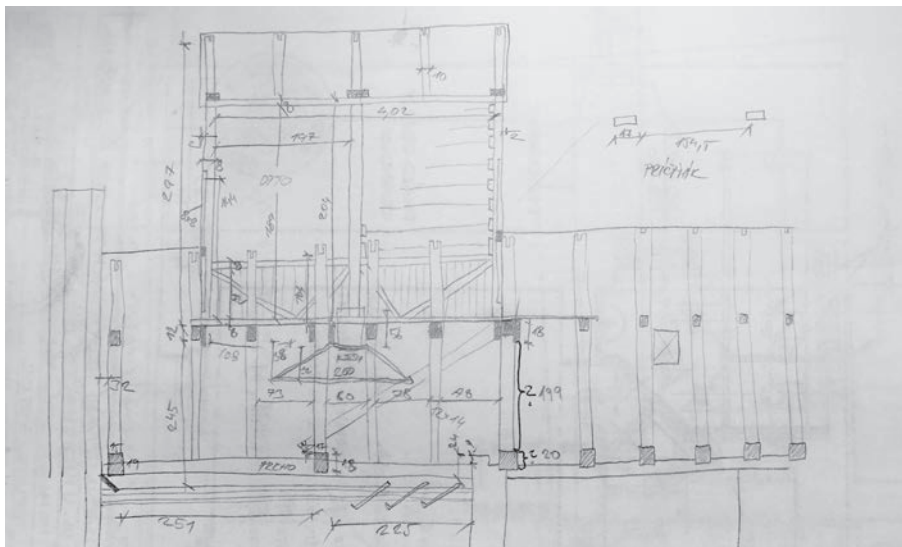
4.7 Terénní náčrt podélného řezu sušárnou chmele v Siřemi č. p. 5, autor: David Skalický 2017.
