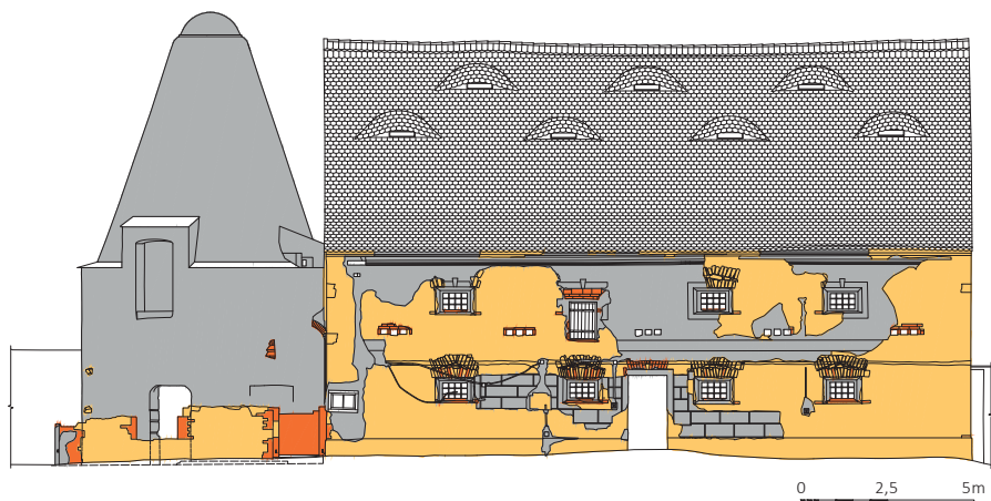
2.12 Analýza západního průčelí sušárny v Rybňanech, p. č. 10/3, autoři: Jan Horák, David Skalický 2018.
