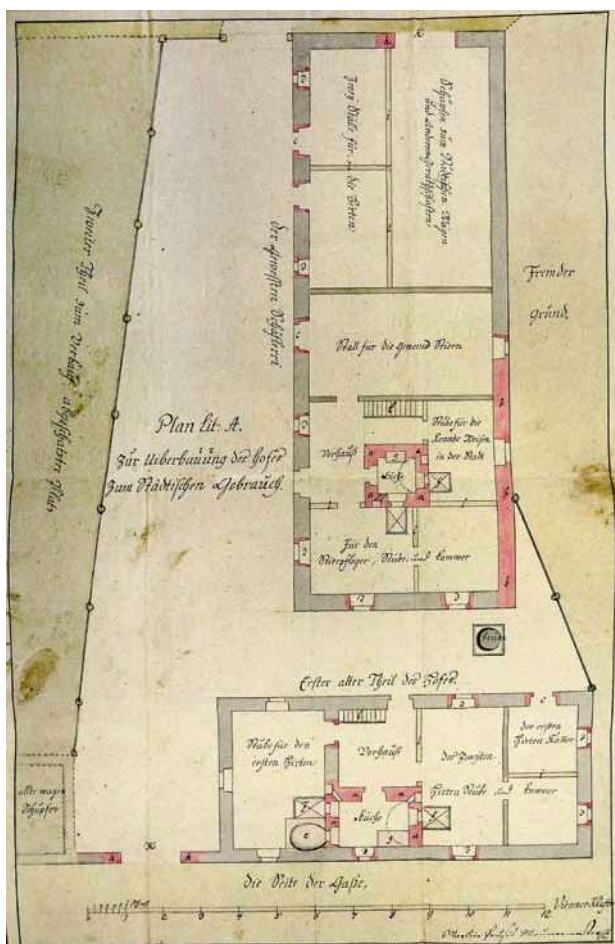
Obr. 1. Martin Prusík: Plan lit. A. Plán stavebních adaptací v obecním dvoře v Kralovicích. Rysováno na papíře, grafické měřítko (vídeňské sáhy). 1795. Signováno. (Státní okresní archiv Plasy, reprofoto P. Vlček, 2016)
