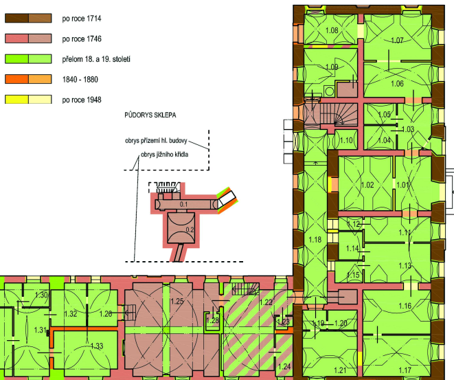
HAJANY - ZÁMEK, PŘÍZEMÍ A SKLEP. ETAPY STAVEBNÍHO VÝVOJE
